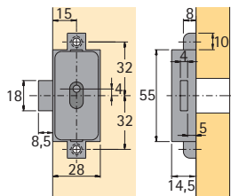
Dornmaß 15 mm, zum Einpressen
