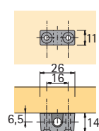
Stangenführung, zum Anschrauben
