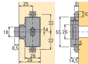
Dornmaß 25 mm, zum Einpressen
