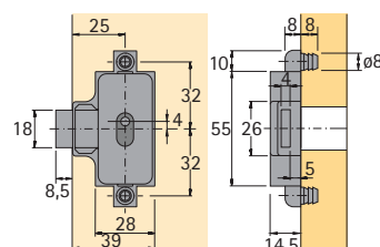
Dornmaß 25 mm, zum Einpressen
