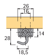
Schließhaken re/li, zum Anschrauben
